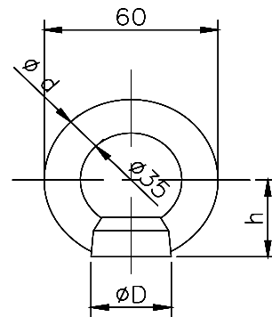
강도계산 형상
